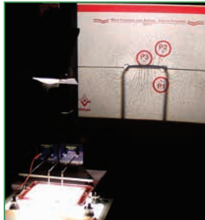
Magnetic field generated by a circular coil (on the overhead projector) / Campo magnético generado por una bobina circular (sobre el retroproyector)
