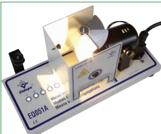
Observing the effect of convection currents / Observación del efecto de las corrientes de convección
