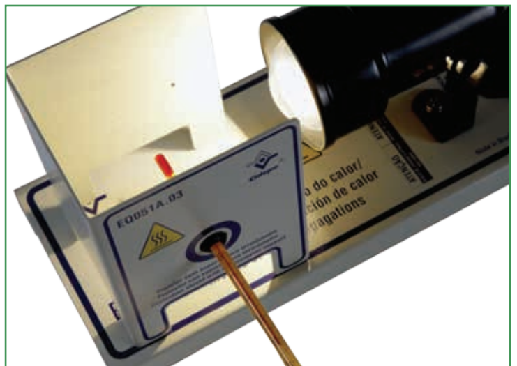
Heating a thermometer bulb by irradiation / Calentamiento del bulbo del termómetro por irradiación
