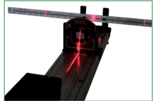
Diffraction and interference with a laser source / Difracción e interferencia con la fuente láser
