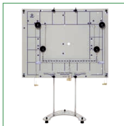
Mechanical advantage of the crossbeam (EQ032G) / Ventaja mecánica del travesaño (EQ032G)
