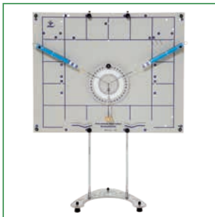
Competing forces at 120° (EQ032E, EQ032G) / Fuerzas concurrentes a 120° (EQ032E, EQ032G)
