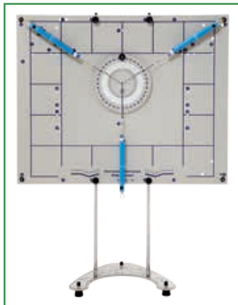
The action of competing forces (EQ032E, EQ032G) / Acción de fuerzas concurrentes (EQ032E, EQ032G)
