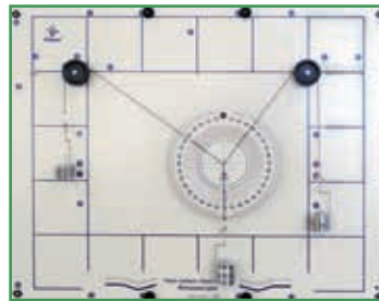
Decomposition of forces, with pulleys (EQ032E, EQ032G) / Descomposición de fuerzas, con roldanas (EQ032E, EQ032G)
